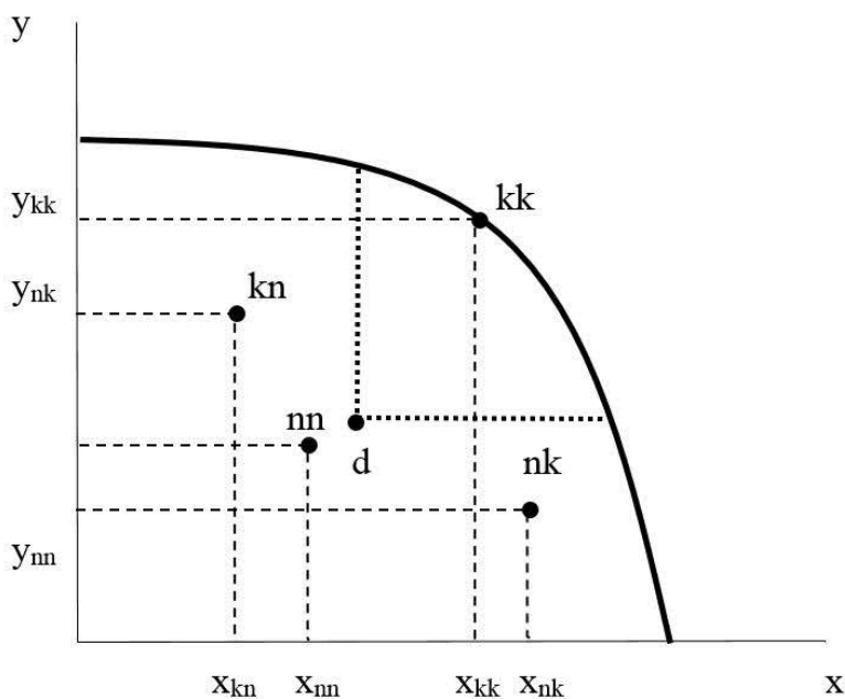
Obrázek č. 4: Rozšíření Nashova vyjednávacího problému o čtyři krajní alternativy
