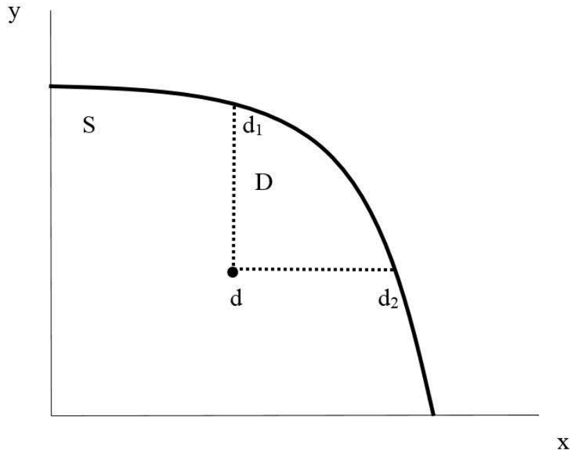
Obrázek č. 1: Základní typ Nashova vyjednávacího problému
