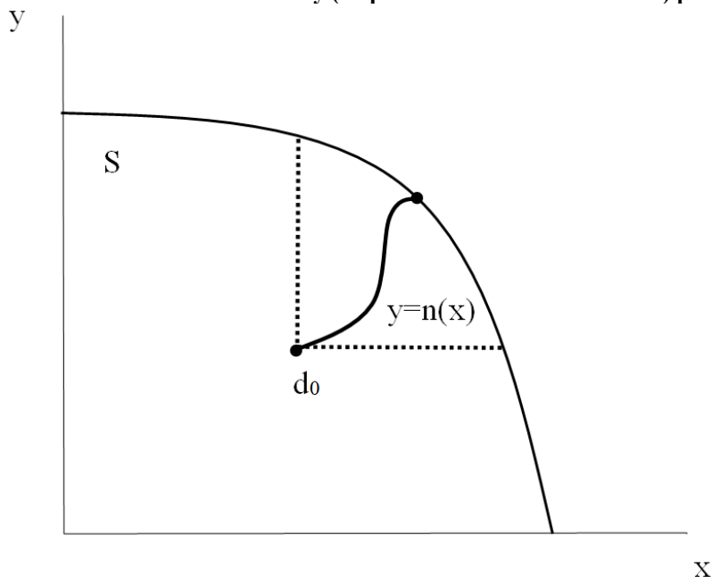
Obrázek č. 7: Funkce neutrality (resp. množina neutrálních bodů) pozičního investování
