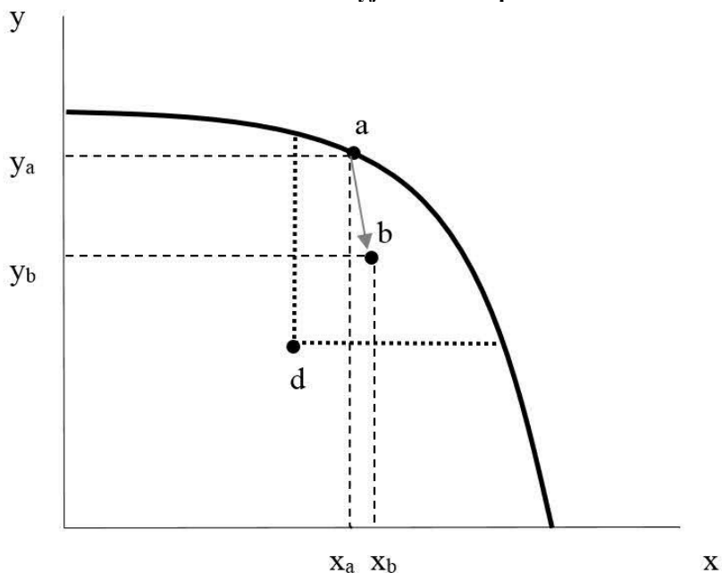
Obrázek č. 3: Nashův vyjednávací problém s více body (typ "hrozba stávkou")
