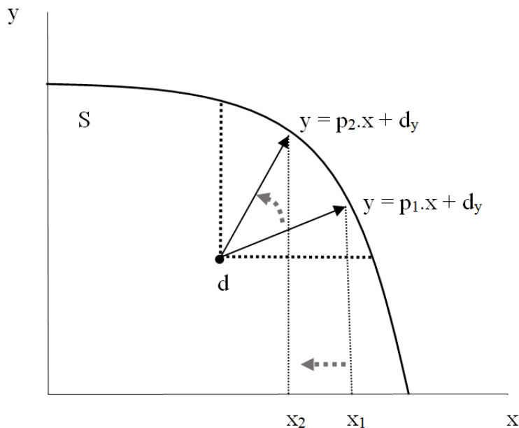
Obrázek č. 9: Interpretace změny sklonu linie pozičního investování
